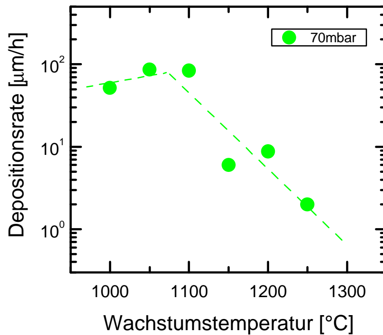
Abb. 5.10 Verlauf der GaN Depositionsrate über T für f_{\text{NH}_3} = 25 sccm und p = 70 mbar.
