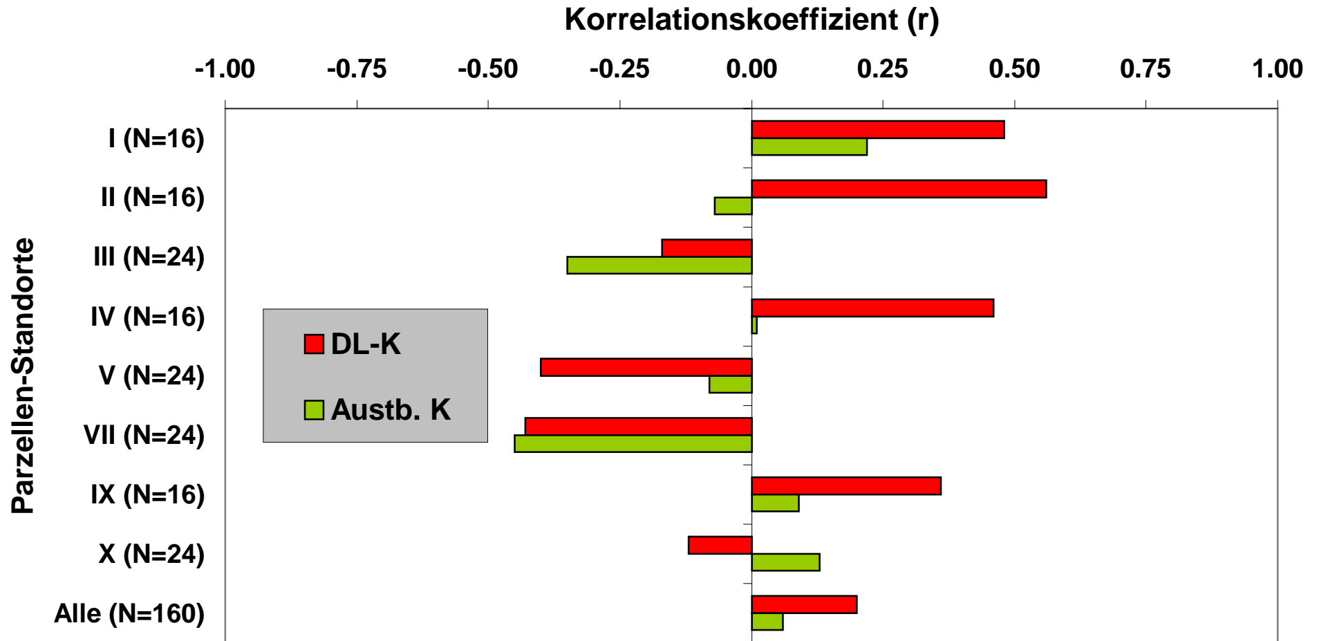
Abb. 20: Beziehungen zwischen der EUF-80°C-K-Fraktion und anderen K-Fractionen in den Böden der Parzellen-Standorte im Hess. Ried (Unberegnete Parzellen, Oberboden 0-30cm)
