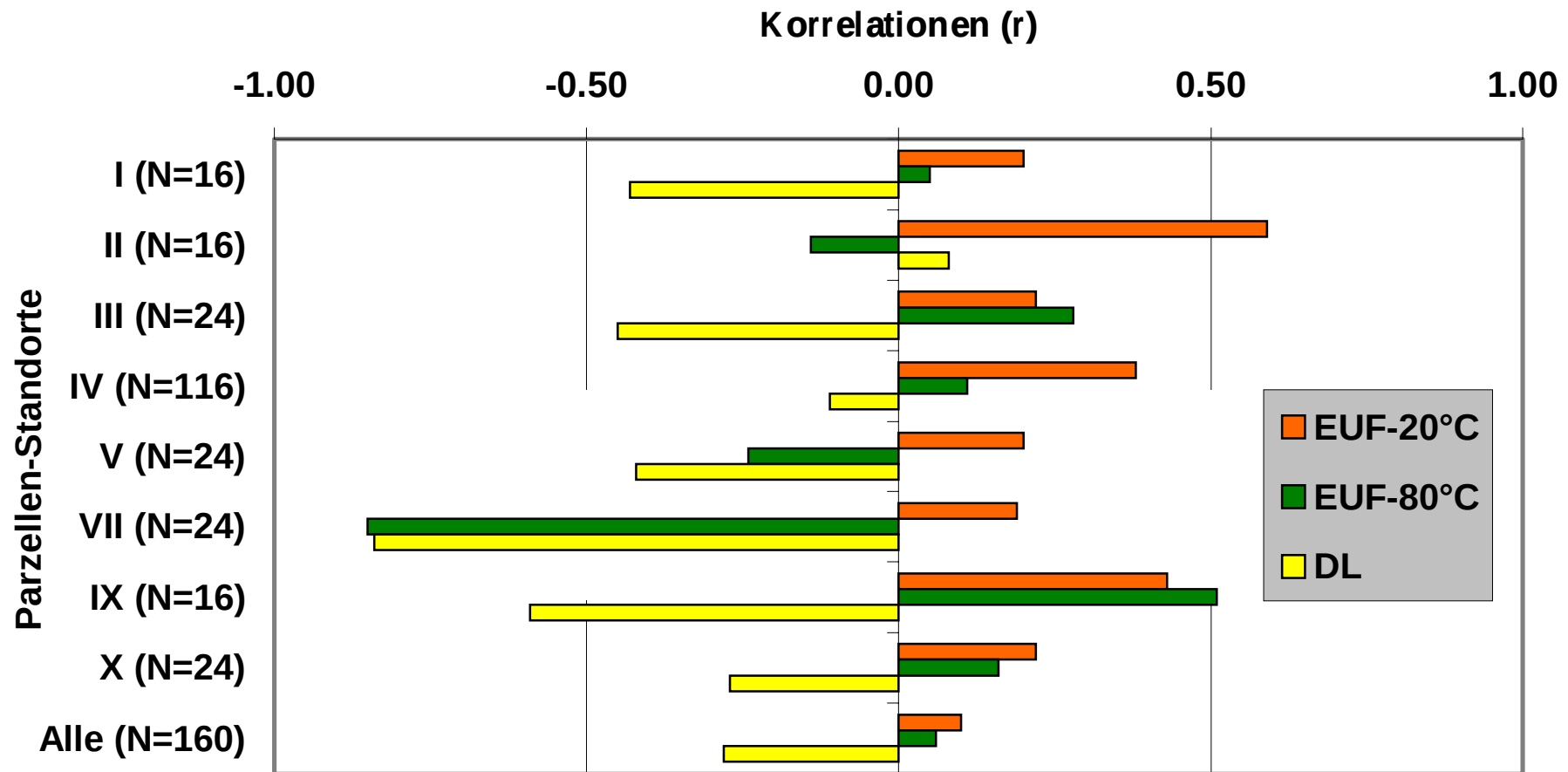
Abb. 23: Beziehungen zwischen einigen Phosphat-Fractionen im Boden (Frühjahr) und dem So.-Weizen-Ertrag (dt'ha -1 Korn) (Hessisches Ried - Unberegnet, Versuchsperiode 1981-1988)
