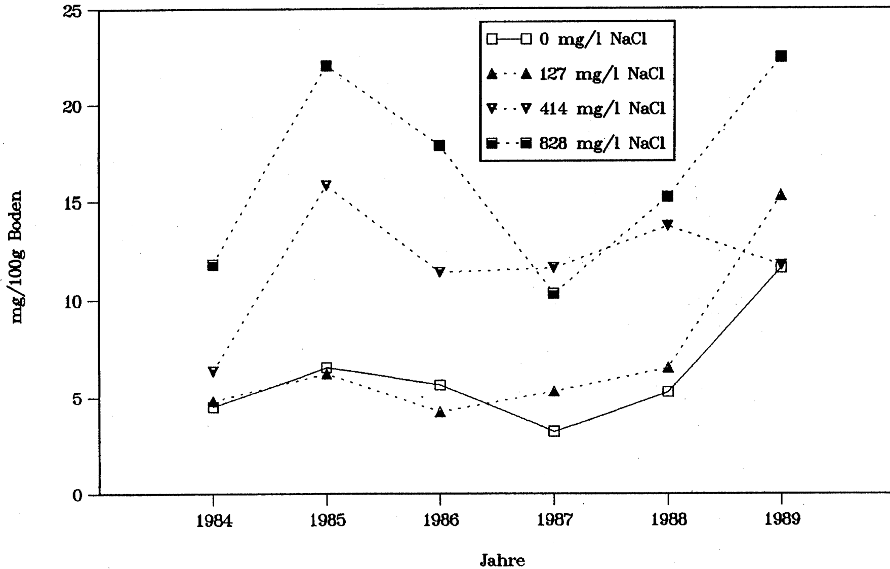
Abb. 24: Der Na-Gehalt (EUF-Gesamt) im Boden von Salinitätsversuch III (Alt) im Verlauf der Jahre
