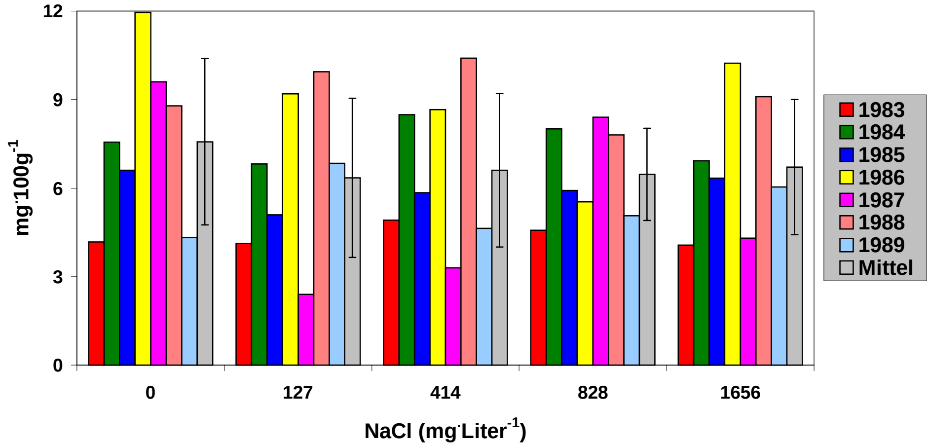
Abb. 29: Der NaCl-Effekt auf das durch die EUF-Methode insgesamt zu extrahierende Phosphat im Boden von Sal.-Versuch V (Alt)
