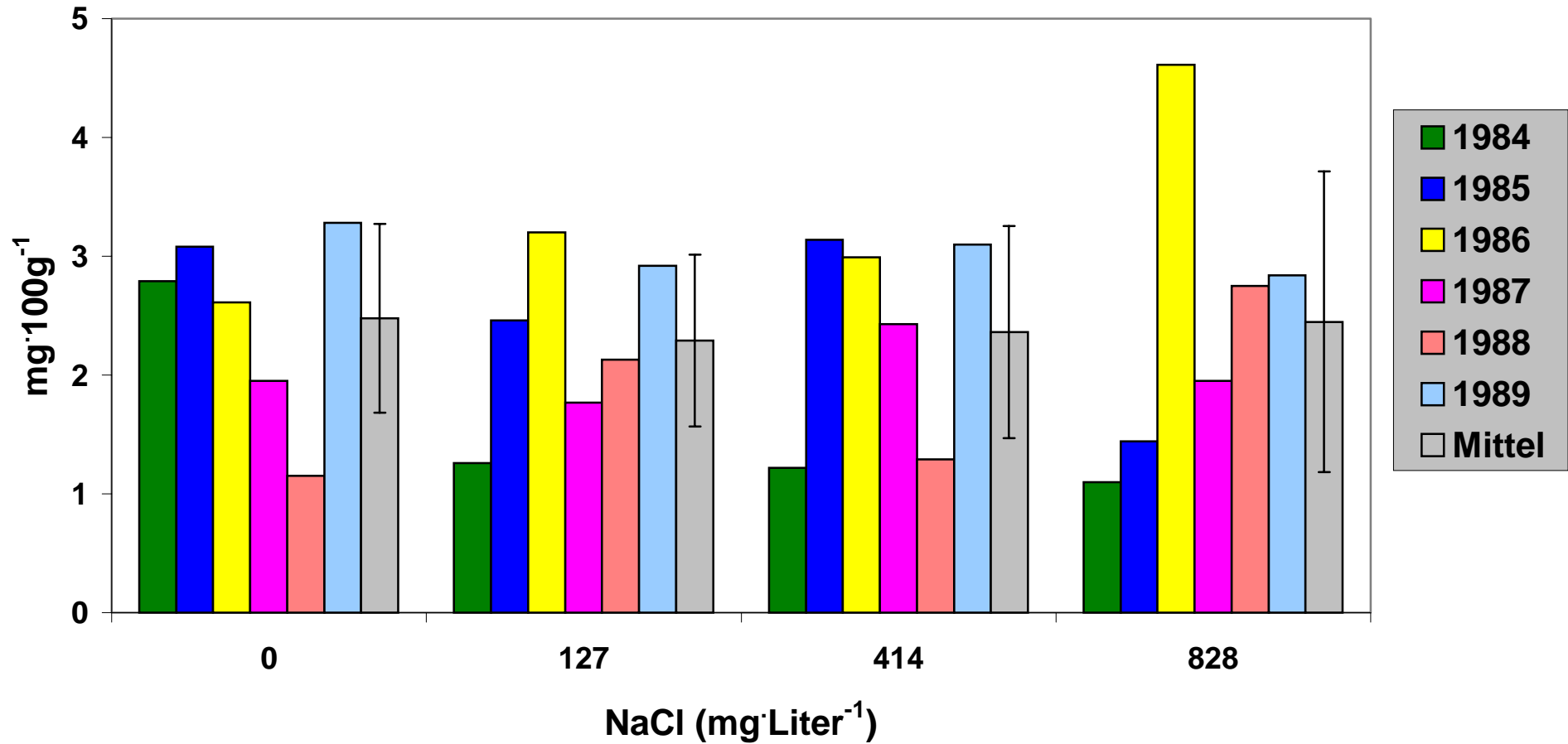
Abb. 31: Der NaCl-Effekt auf das durch die EUF-Methode insgesamt zu extrahierende Nitrat im Boden von Sal.-Versuch III (Alt)
