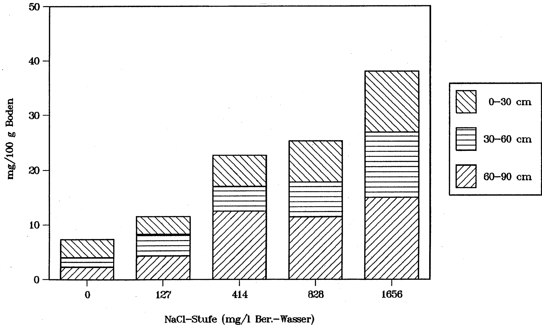
Abb. 36: Verteilung des durch die EUF-Methode insgesamt zu extrahierenden Natriums in unterschiedlichen Bodentiefen von Salinitätsversuch V (Alt)
