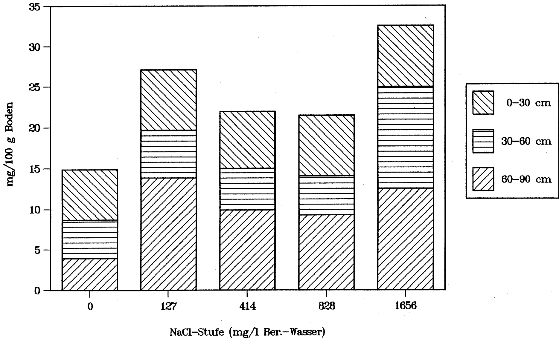
Abb. 37: Verteilung des durch die EUF-Methode insgesamt zu extrahierenden Chlorids in unterschiedlichen Bodentiefen von Salinitätsversuch V (Alt)
