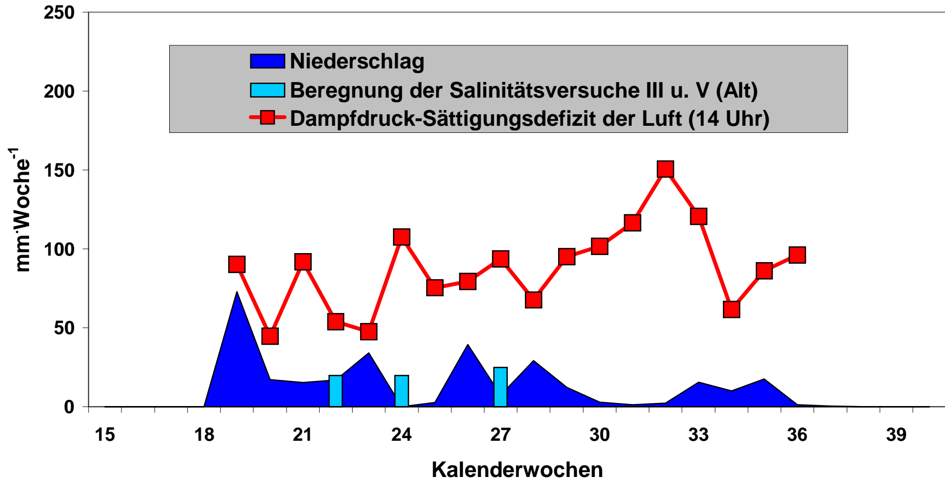
Abb. 40: Wochensummen des Dampfdruck-Sättigungsdefizits der Luft (14°) und des Niederschlags in der Hauptberechnungsperiode 1988
