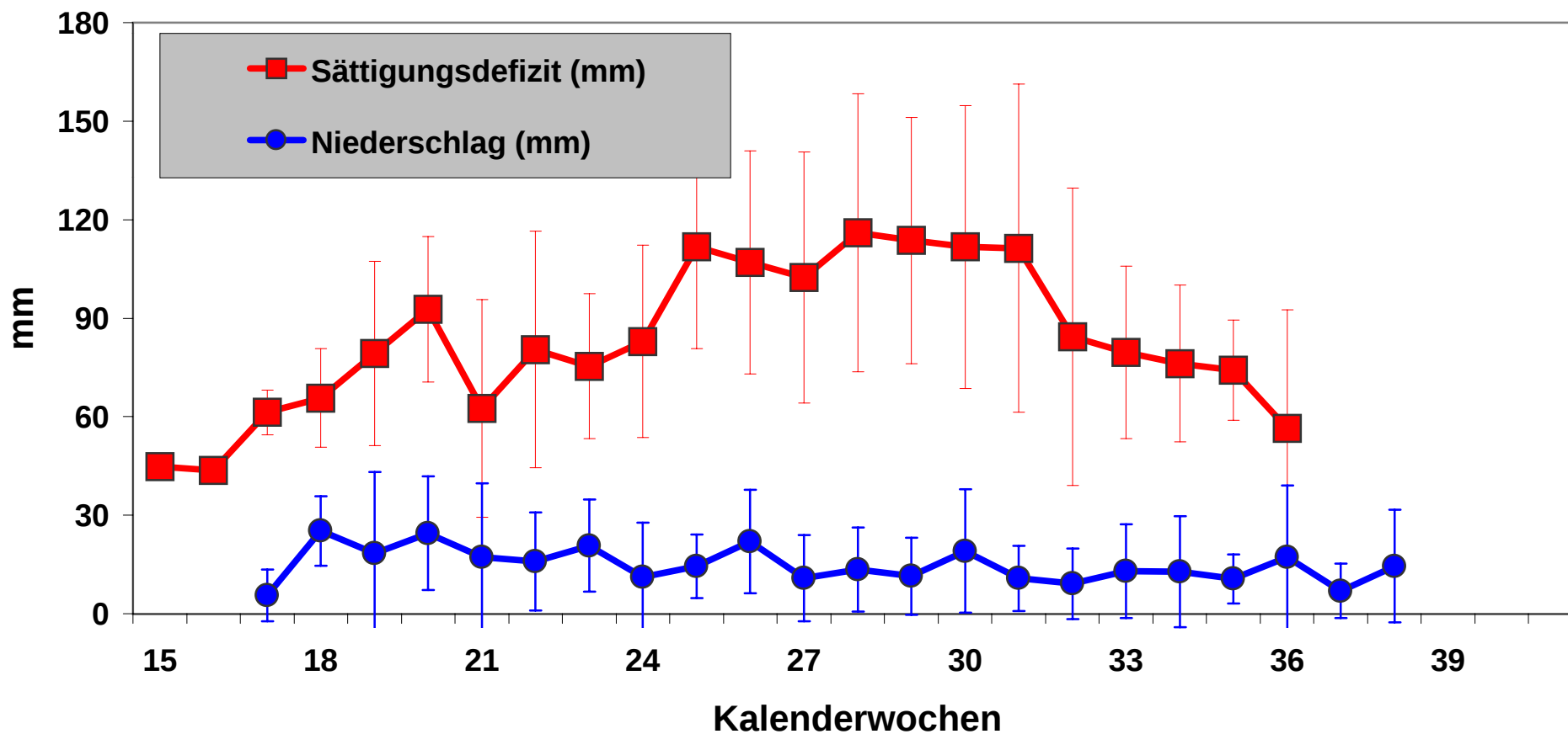
Abb. 7: Mittlere Wochensummen des Dampfdruck-Sättigungsdefizits der Luft (14°) und des Niederschlags während der Hauptberechnungsperiode in den Jahren 1981-1992 im mittleren Hessischen Ried
