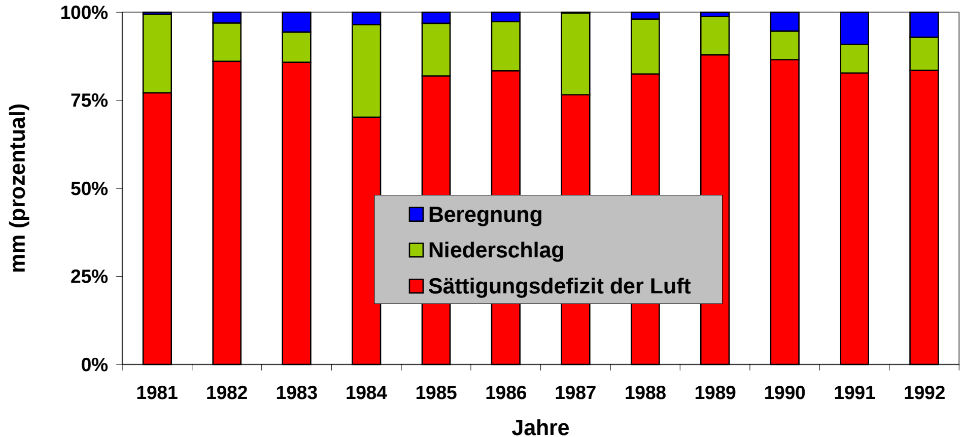
Abb. 9-III: Gegenüberstellung der mittleren Wochensummen des Dampfdruck-Sättigungsdefizits der Luft, des Niederschlags und der mittleren Beregnung zu Feldgemüse während der Hauptberegnungsperiode der Jahre 1981-1992 im Hessischen Ried
