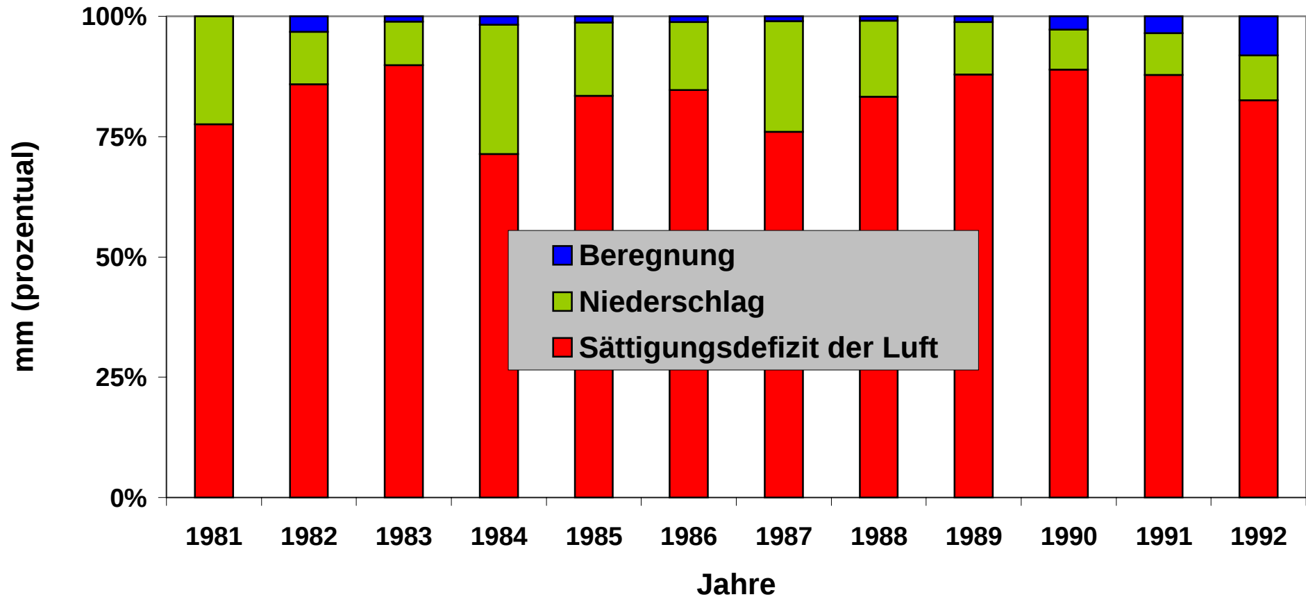
Abb. 9-I: Gegenüberstellung der mittleren Wochensummen des Dampfdruck-Sättigungsdefizits der Luft, des Niederschlages und der Beregnung zu So.-Weizen während der Hauptberegnungsperiode der Jahre 1981-1992 im Hessischen Ried
