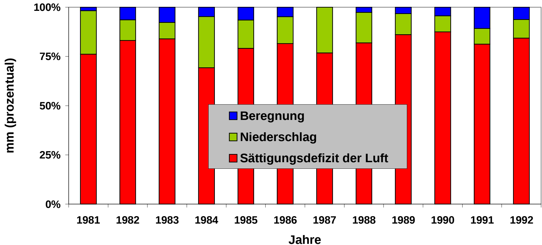
Abb. 9-II: Gegenüberstellung der mittleren Wochensummen des Dampfdruck-Sättigungsdefizits der Luft, des Niederschlags und der mittleren Beregnung zu Zuckerrüben während der Hauptberegnungsperiode der Jahre 1981-1992 im Hessischen Ried
