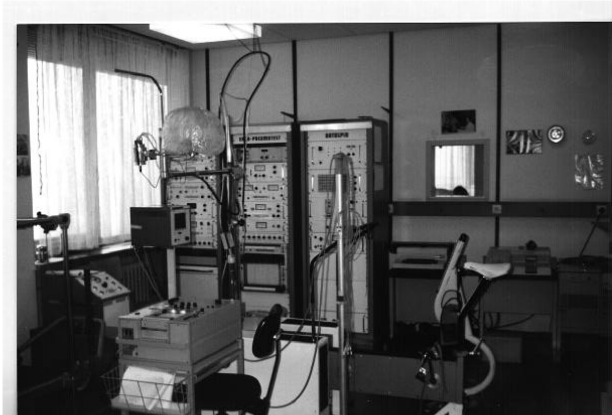
Abb. 12: Kompletter spirometrischer Meßplatz der Firma E. Jaeger/ Würzburg an der Professur für Sportmedizin der Justus-Liebig- Universität Gießen zur körperlichen, kardiozirkulatorischen und kardiorespiratorischen Funktionsdiagnostik im offenen System. Die Registrierung der Ventilationsgrößen erfolgte fortlaufend pneumotachographisch; Messung der Sauerstoff- und Kohlendioxydkonzentrationen in Volumen % nach der Wärmeleitmethode.
