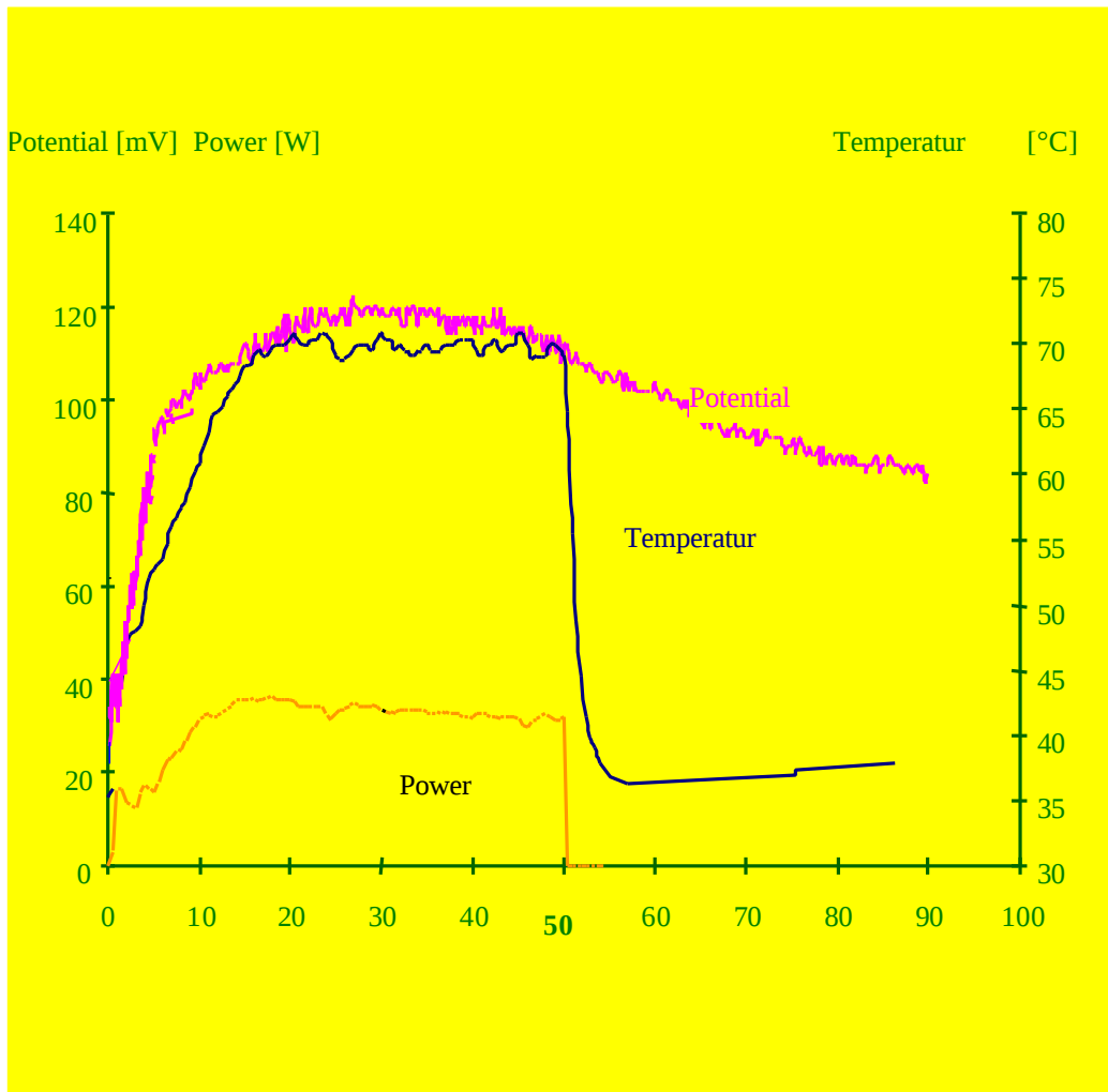
Abb. 5: Auf der Abszisse ist die Zeit in Sekunden aufgetragen. Beziehung zwischen der Katheterspitzen-Temperatur ( ^{\circ}\text{C} ), gemessenem Potential (mV) und Hochfrequenzenergie(HF)-Abgabe über 50 Sekunden. Keine Vaporisation.
