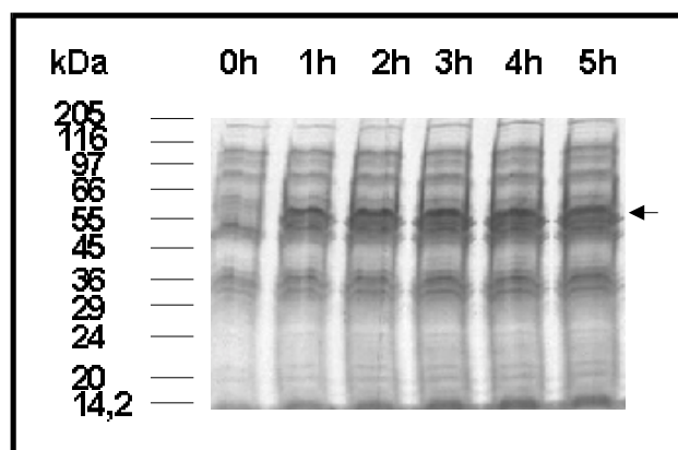
Abb. 35: Ermittlung der optimalen Expressionsbedingungen für FP-1
