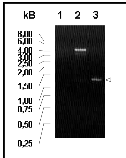
Abb. 34: Vergleich der isolierten Plasmide mit dem ursprünglichen PCR-Produkt der FP-1
