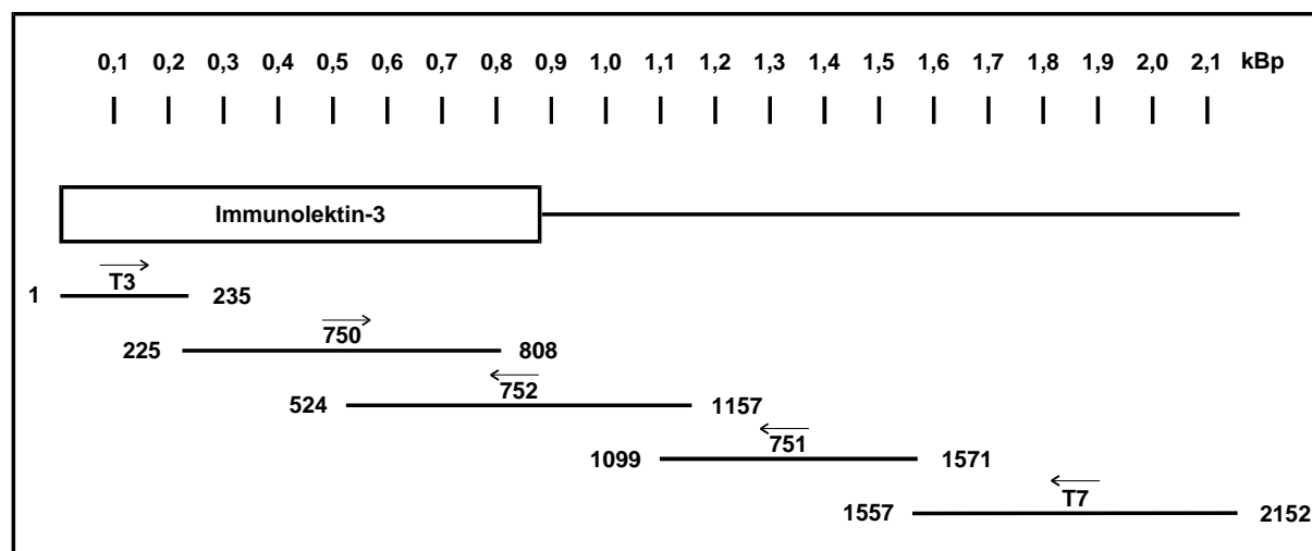
Abb. 19: Strategie zur Sequenzierung der ursprünglich isolierten cDNA des IML-3
