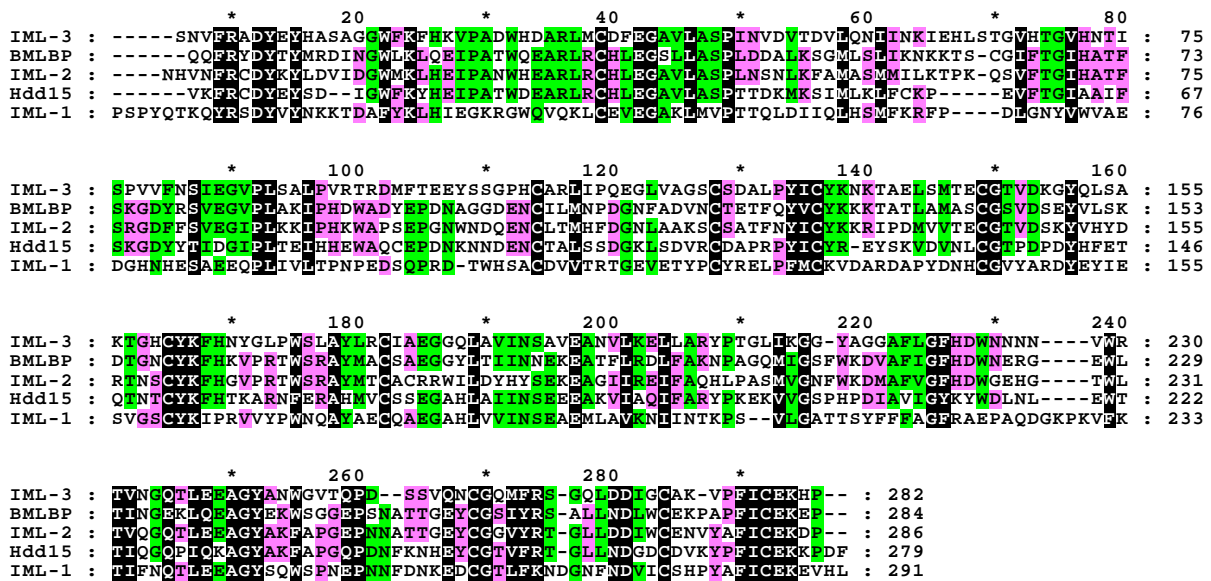
Abb. 20: Alignment von IML-3 mit Calcium-abhängigen Lektinen, die zwei CRDs besitzen
