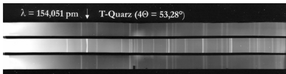
Abbildung 27: Pulveraufnahme von \text{Tl}_2\text{MoF}_6
