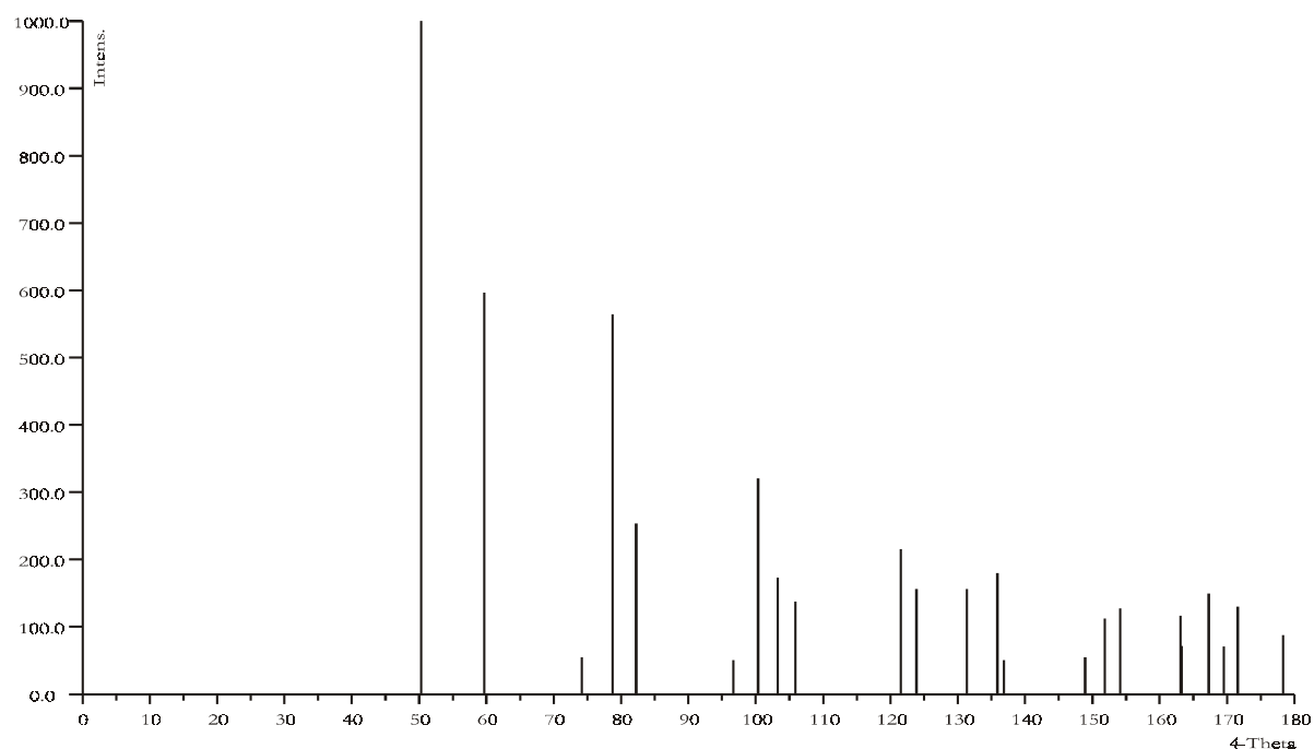
Abbildung 22: Simulation einer Pulveraufnahme von \text{Ti}_2\text{RuF}_6
