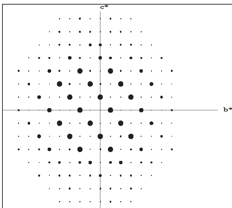
Abbildung 11: Reziprokes Gitter der 1\ k\ l -Ebene von \text{Tl}_2\text{PtF}_6
