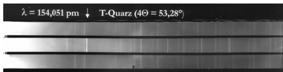
Abbildung 34: Pulveraufnahme von \text{Tl}_2\text{TaF}_6
