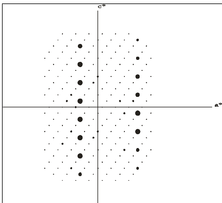
Abbildung 87: Reziprokes Gitter der h\ 1\ l -Ebene
