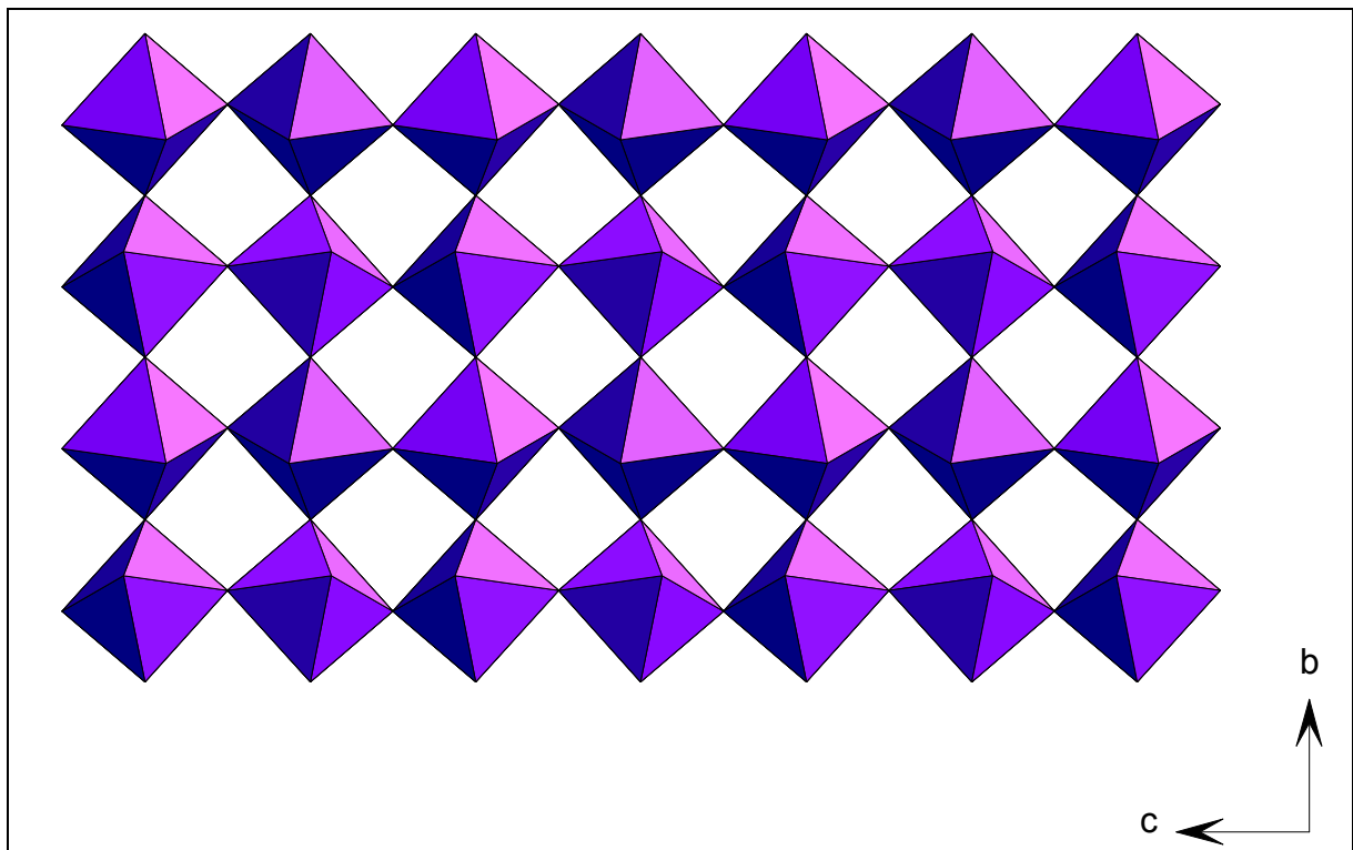
Abbildung 46: Verknüpfung der \text{TlF}_6 -Oktaeder zu \text{TlF}_{4/2}\text{F}_2 -Schichten
