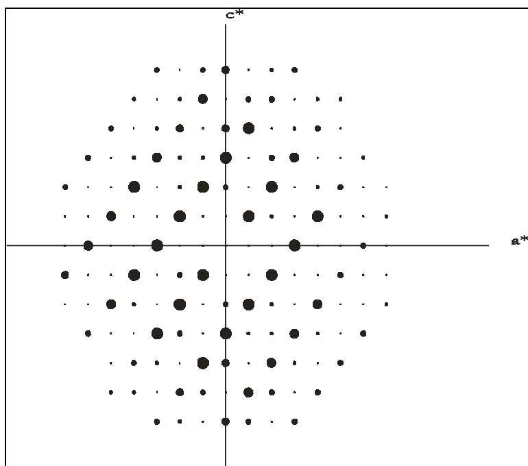
Abbildung 14: Reziprokes Gitter der h\ 0\ l -Ebene von \text{Tl}_2\text{ReF}_6
