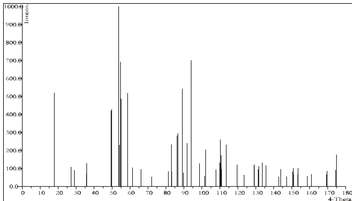
Abbildung 65: Simulation einer Pulveraufnahme von \text{Rb}_2\text{Zr}_3\text{F}_{12}\text{O}
