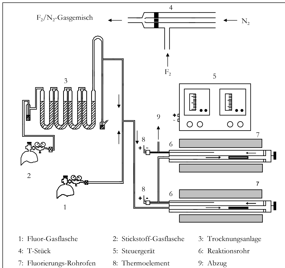
Abbildung 1: Fluorierungsöfen
