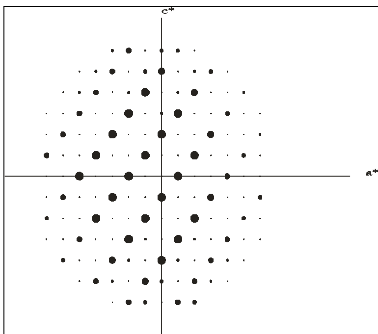
Abbildung 15: Reziprokes Gitter der h\ l\ l -Ebene von \text{Tl}_2\text{ReF}_6
