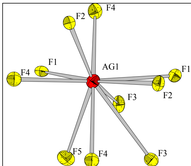
Abbildung 96: Koordinationspolyeder um Ag1
