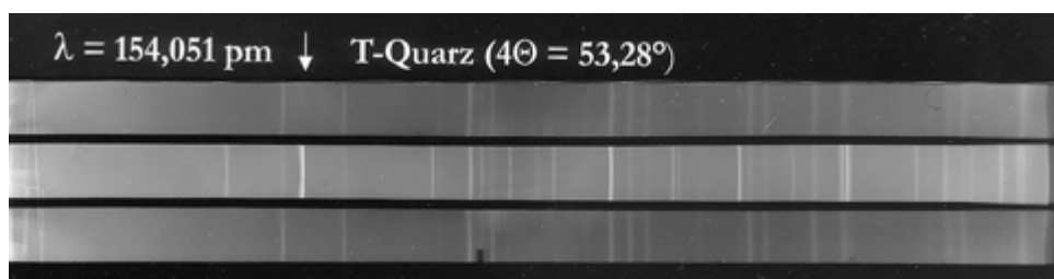
Abbildung 23: Pulveraufnahme von \text{Ti}_2\text{RuF}_6
