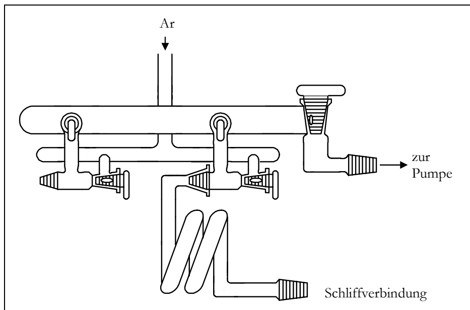
Abbildung 2: Verteilerapparat
