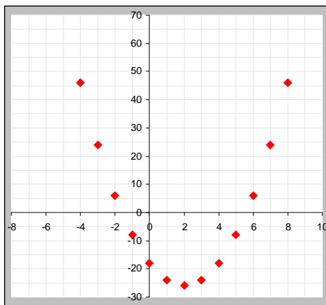
Abb. 16: Die Z-Funktion f(n) = 2n^2 - 8n - 18 und deren Differenzenfunktion
