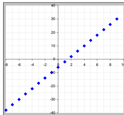
Abb. 17: Die Z-Funktion f(n) = 2n^2 - 8n + 12 und deren Differenzenfunktion
