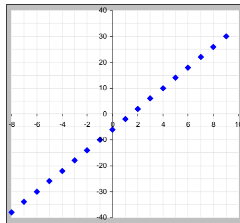
Abb. 16: Die Z-Funktion f(n) = 2n^2 - 8n - 18 und deren Differenzenfunktion
