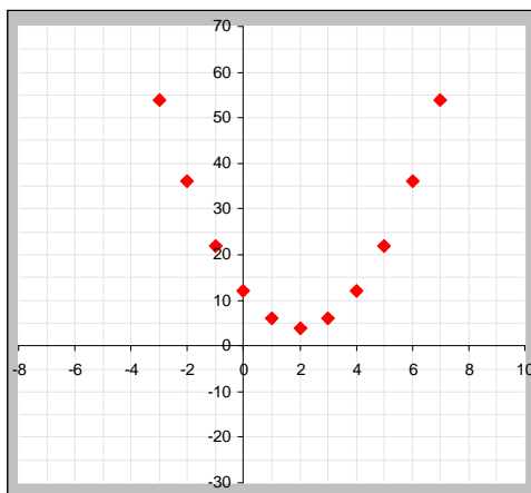
Abb. 17: Die Z-Funktion f(n) = 2n^2 - 8n + 12 und deren Differenzenfunktion
