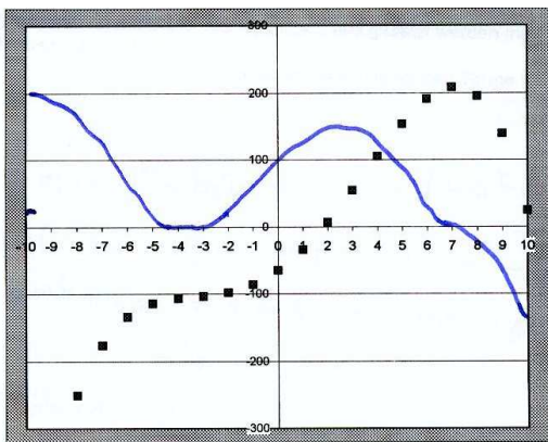
Abb. 85: Aufgabe 5 – Qualitativ richtige Lösung (Studierender II6)
