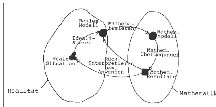
Abb. 19: Der Modellbildungsprozess (aus Blum & Törner 1983, S. 248)
